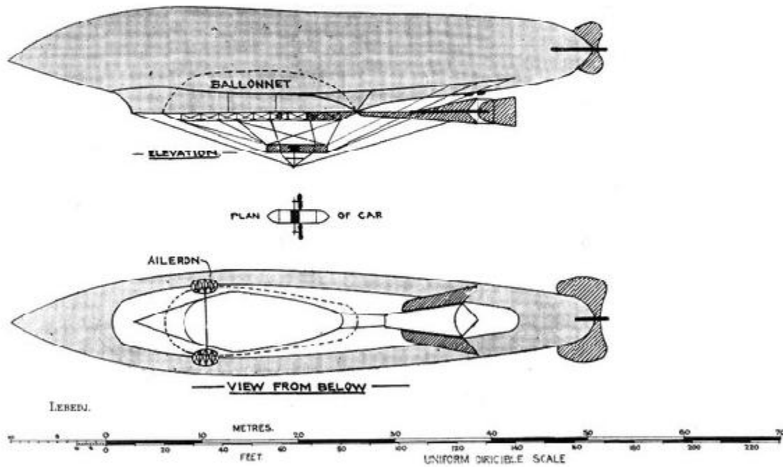
Lebedj. Uniform Dirigible Scale.
